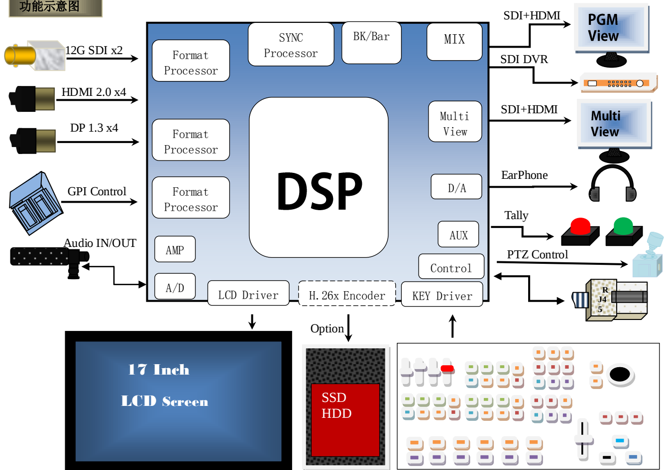
功能示意图
