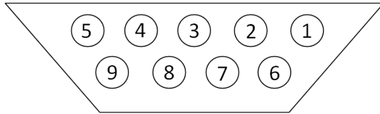
DB-9Pin 接口引脚定义图（母头）
